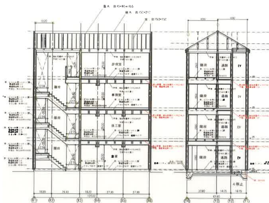
図 1-8 診療所 耐火木造 4階 断面図
